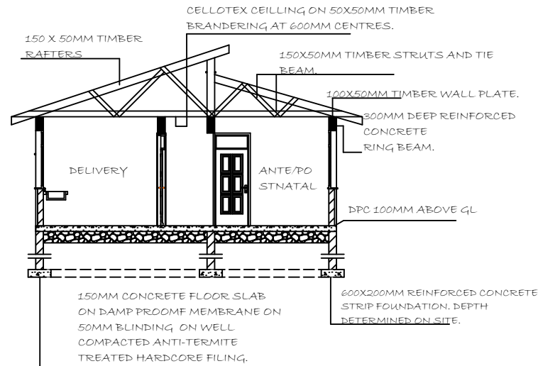
SEC'A-A
